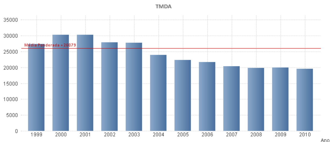
Figura 6 – Evolução do TMDA 1999-2010
