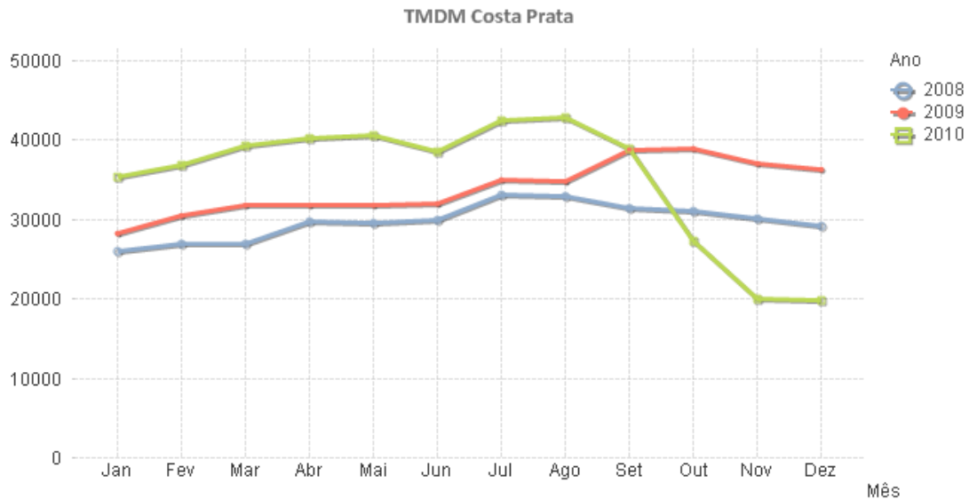
Figura 18 - Variação do TMDM na concessão Costa de Prata (2008-2010)
