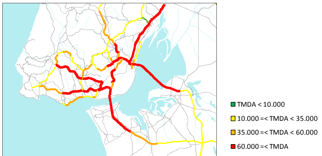
Figura 22 - Fluxos de Tráfego na Área Metropolitana de Lisboa
