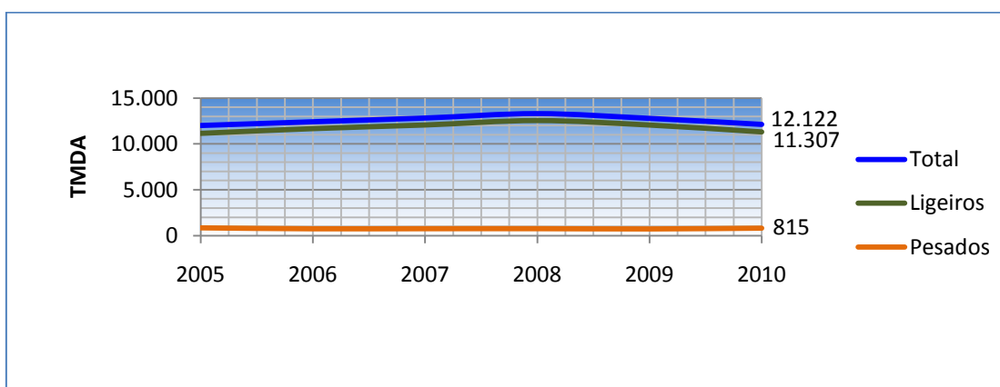
Figura 11 - Evolução do TMDA na A22/E01 Ponte Internacional do Guadiana
