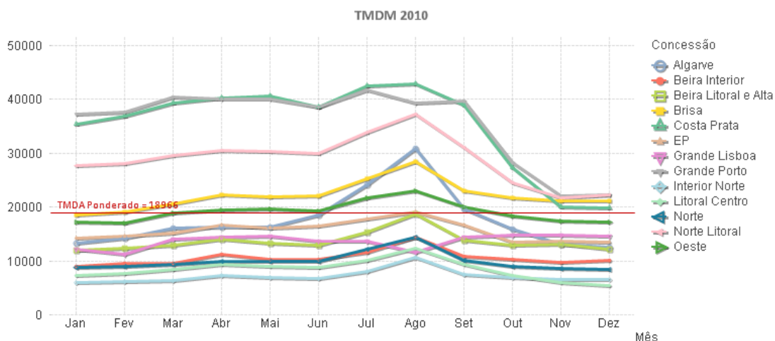
Figura 13 – TMD Mensal 2010 por Concessionária
