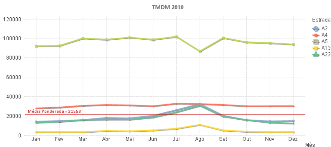
Figura 14 – Variação do Tráfego durante o ano
