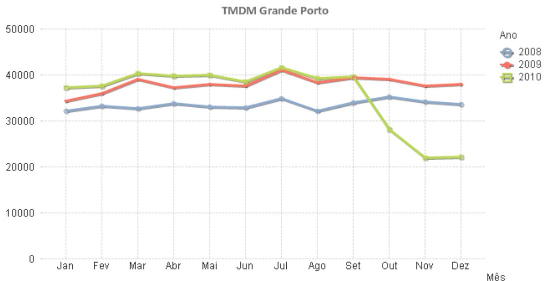
Figura 19 - Variação do TMDM na concessão Grande Porto (2008-2010)
