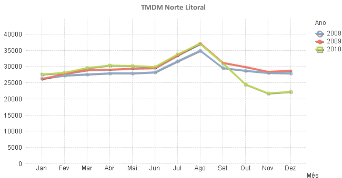
Figura 20 - Variação do TMDM na concessão Norte Litoral (2008-2010)
