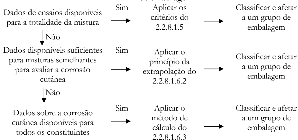
Figura 2.2.8.1.6.1: Abordagem para a classificação e afetação de misturas corrosivas aos grupos de embalagem
