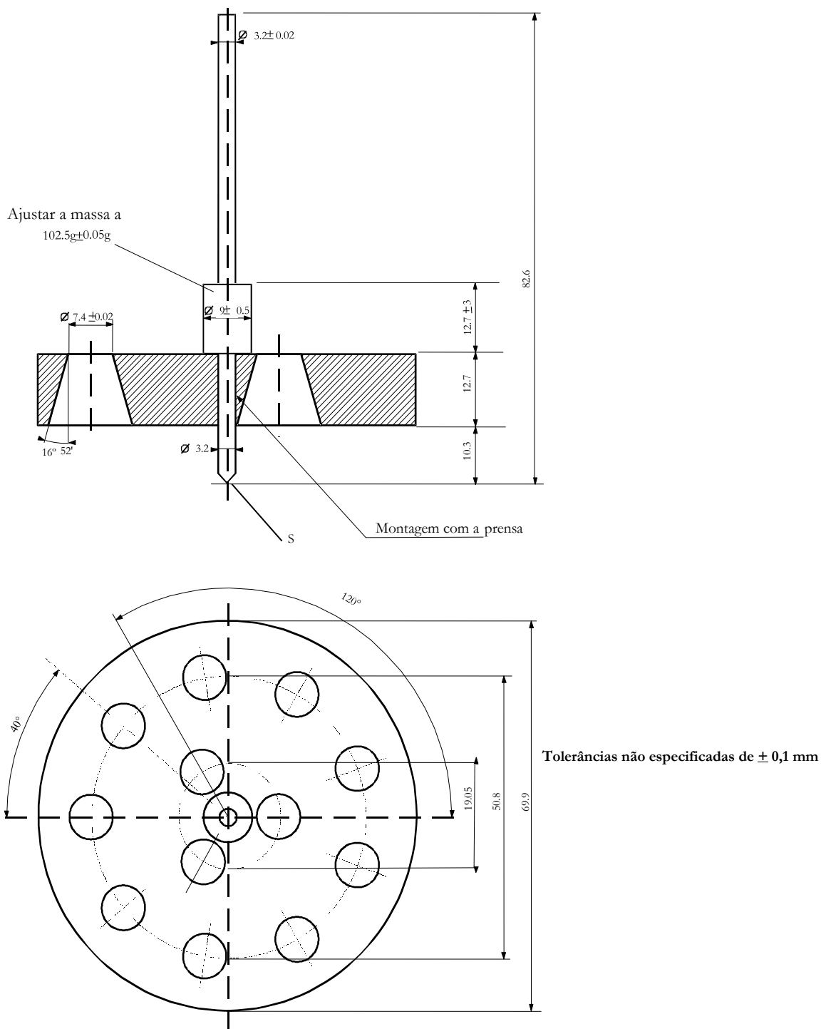
Figura 1 – Penetrómetro
